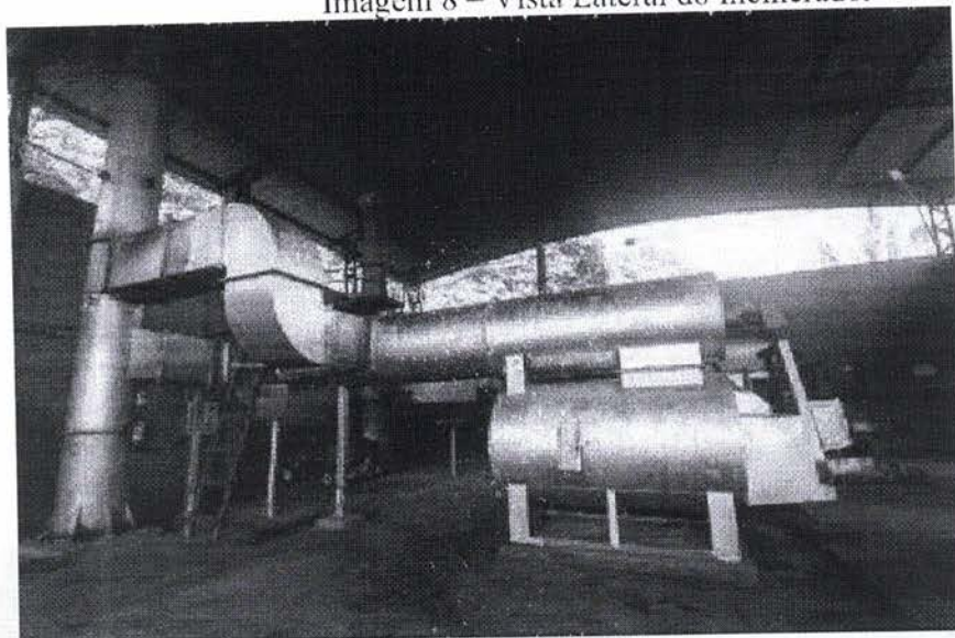
Imagem 8 – Vista Lateral do Incinerador
