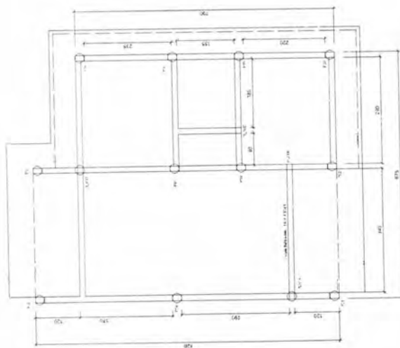
ESQUEMATICO BALDRAMES E VIGAS SUPERIORES
